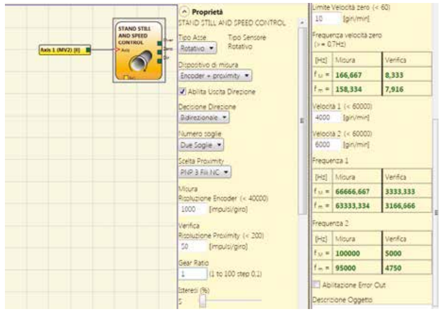
Esempio di configurazione del controllo velocità
