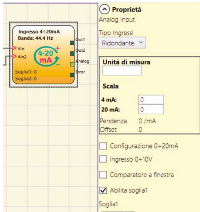
Parametri di configurazione ingressi analogici
