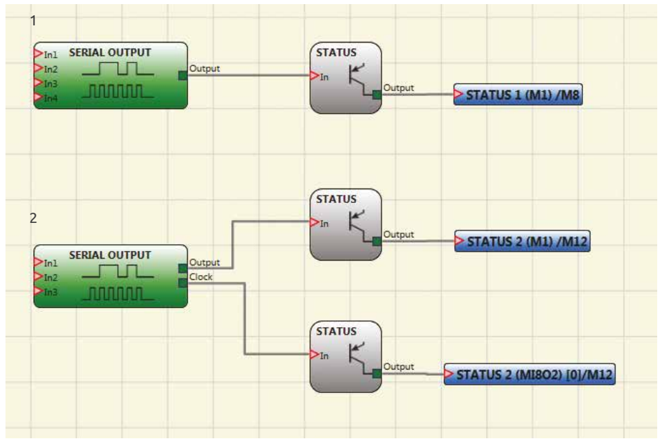
Tipi di collegamento del modulo HM1
