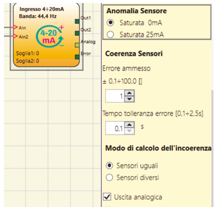
Configurazione dei parametri di coerenza dei sensori per verificare lo stato di funzionamento
