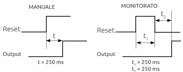
Reset manuale o monitorato
