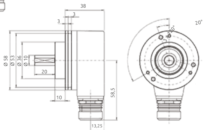
Encoder, albero sporgente con piattina
