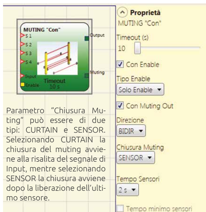
Esempio di configurazione di Muting T contemporaneo
