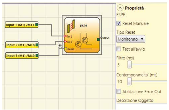
Esempio di configurazioni dell'ESPE
