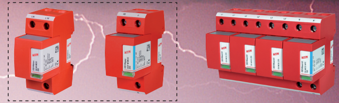
961 120 DEHNbloc M 255 961 101 DEHNgap M 255 951 310 DEHNventil M TT 255
