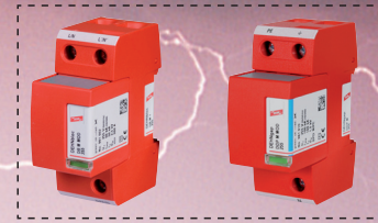
961 120 DEHNbloc M 255 961 101 DEHNgap M 255
